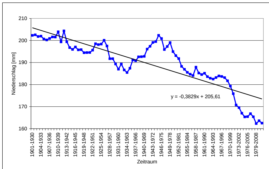
Abbildung 21: 30jährig gleitendes Mittel des Niederschlags in der Vegetationsperiode 1 (April bis Juni) an der Station Görlitz von 1901 – 2010 69
