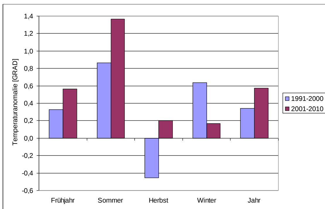
Abbildung 18: Anomalie der Mitteltemperatur in den Dekaden 1991 - 2000 und 2000 - 2010 gegenüber der Referenzperiode 1981 - 1990 im Raum Görlitz 66
