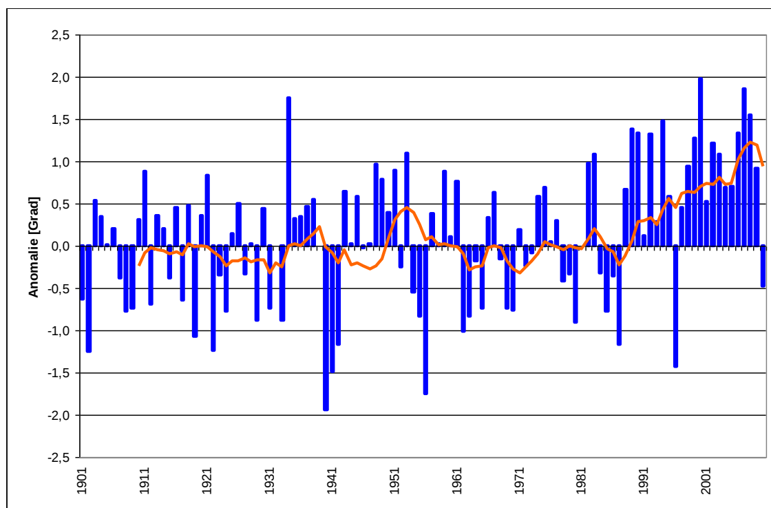
Abbildung 17: Anomalie und dekadische Variabilität der Jahresmitteltemperatur 1901 – 2010 im Raum Dresden (Referenzperiode 1961 - 1990 mit der Jahresmitteltemperatur 8,6 °C für Dresden-Klotzsche) 65
