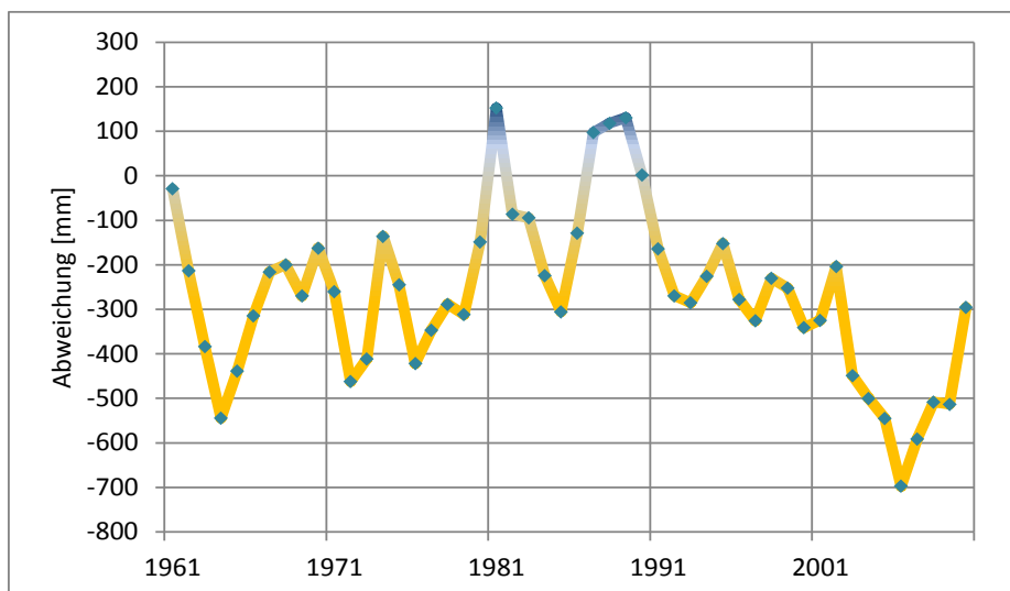
Abbildung 19: Abweichung des kumulierten Jahresniederschlages im Raum Dresden von 1961 bis 2010 im Vergleich zum mittleren kumulierten Jahresniederschlag 1961 - 1990 67
