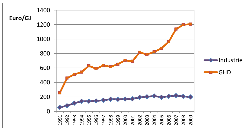
Abbildung 12: Energieproduktivität in Industrie und im Bereich GHD 1991 bis 2009 47,48,49
