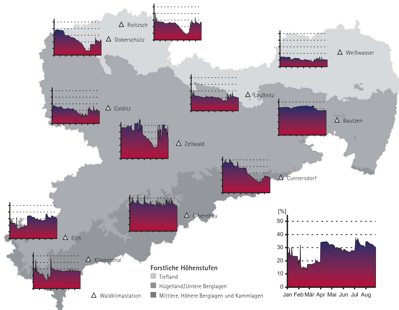
Abb. 3: Verlauf der täglichen Minima der Bodenfeuchte in 30 cm Tiefe an ausgewählten Waldklimastationen
