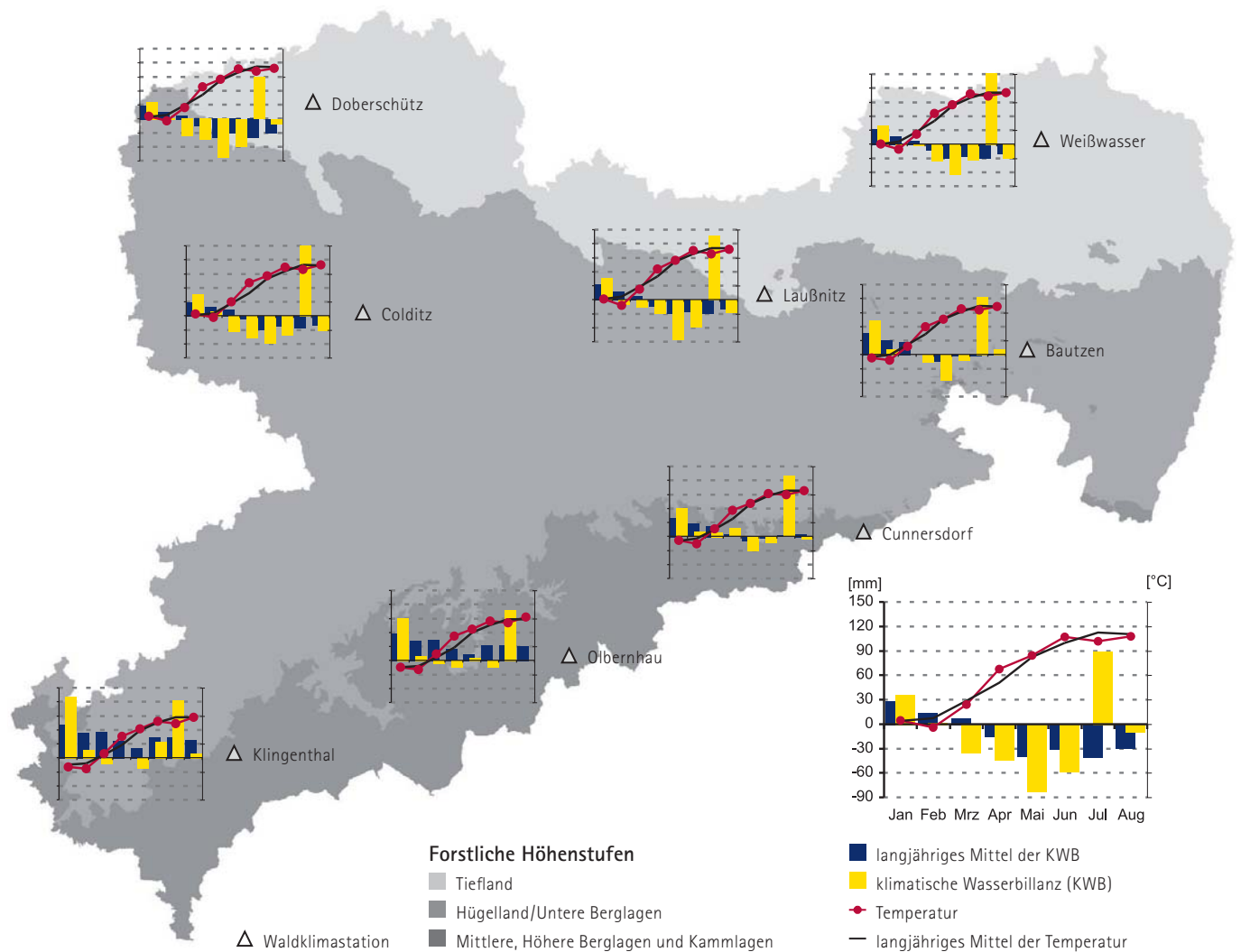
Abb. 2: Monatsmittel der Lufttemperaturen und die klimatische Wasserbilanz von Januar bis August 2011 für ausgewählte Waldstandorte
