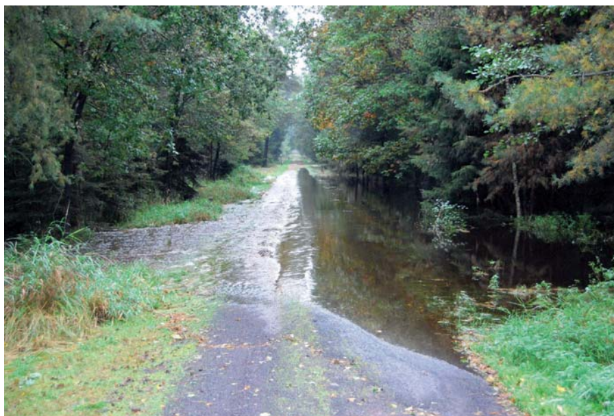
Abb. 4: Intensive Niederschläge führten im Herbst 2010 im Bereich der wassergesättigten Niedermoores in der Laußnitzer Heide zu enormen oberflächlich abfließenden Wassermassen
